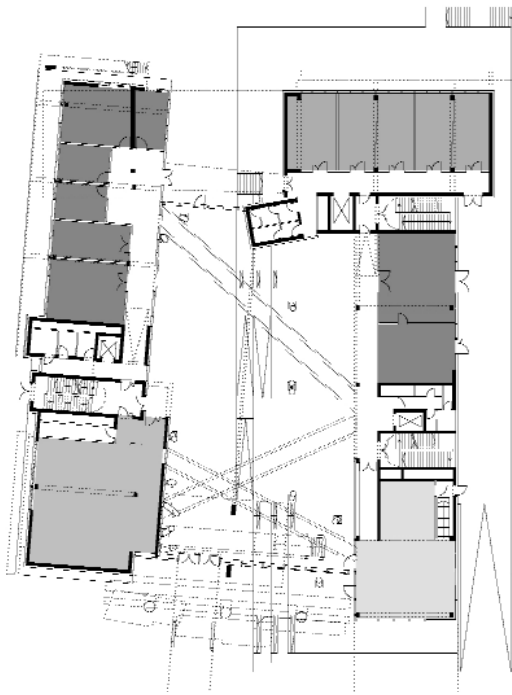
Grundrisse Erdgeschoss, 1. Obergeschoss (oben von links), 2. und 3. Obergeschoss (unten von links)
